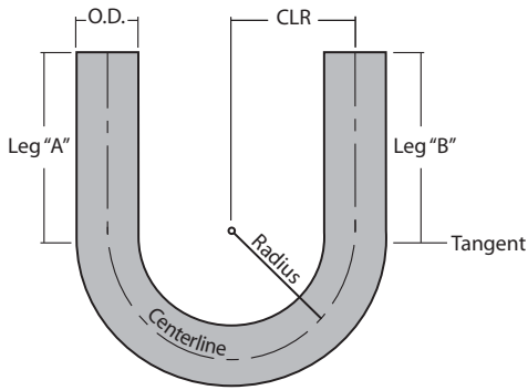
U bend 180°
