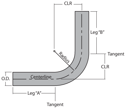
90° Bend
